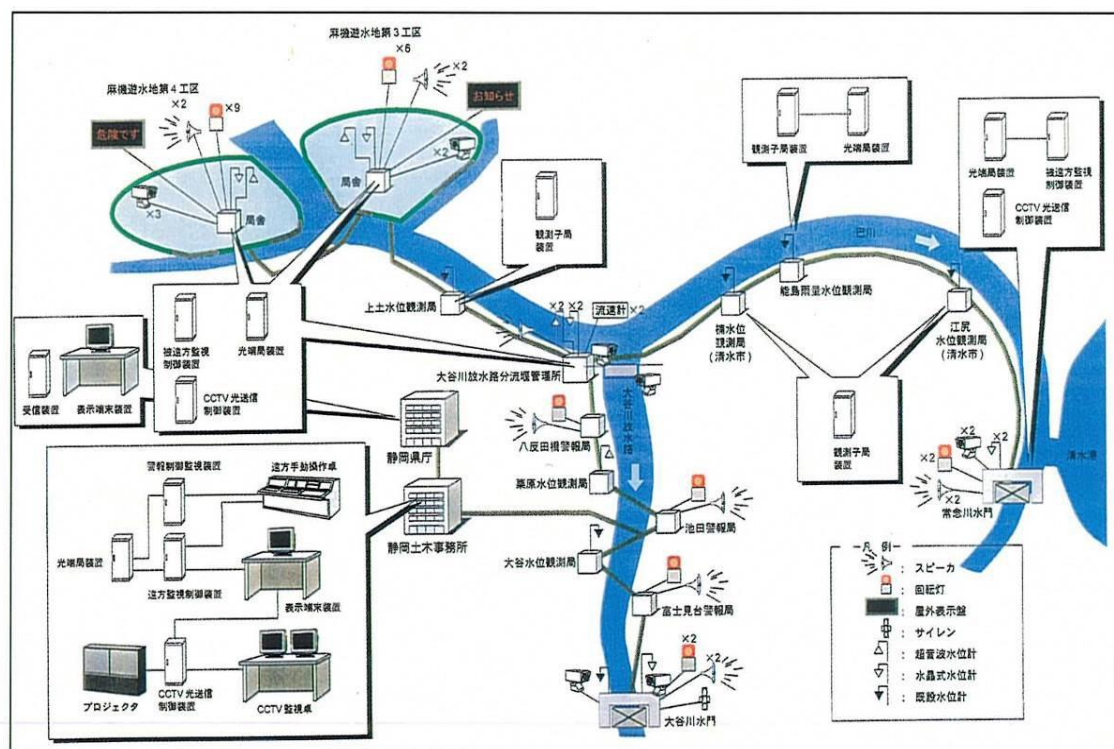
図 2-12 巴川情報管理システム
