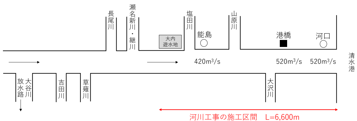
図 4-7 流量配分図
