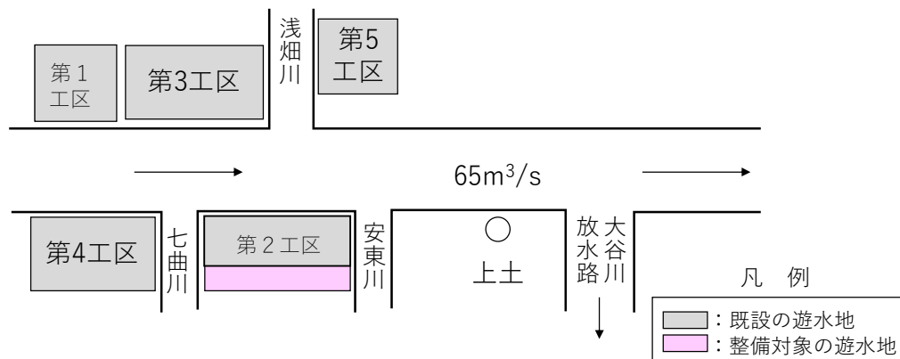
図 4-3 流量配分図
