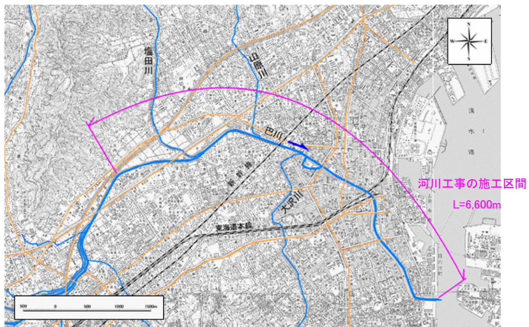
図 4-6 河道掘削の整備箇所
