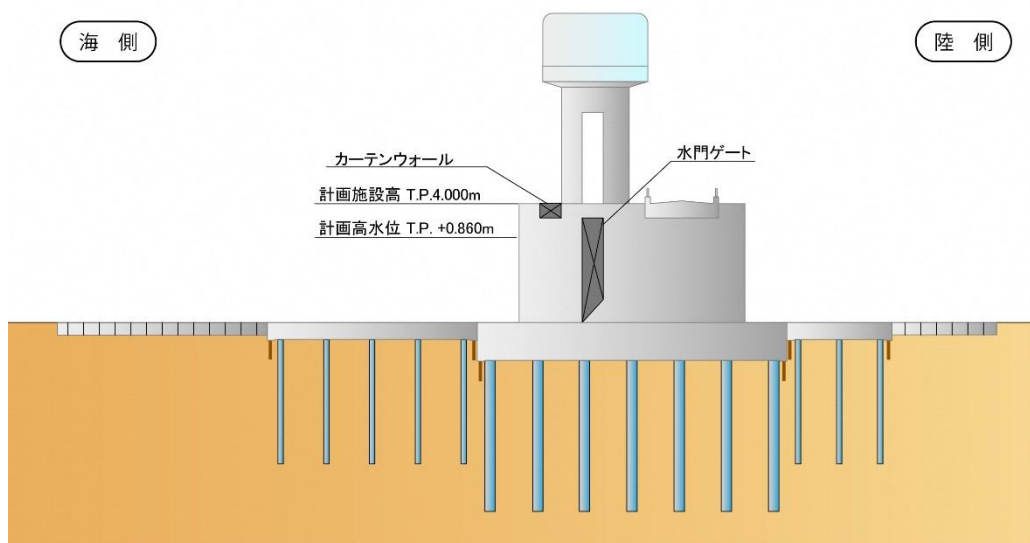
図 4-13 津波対策水門イメージ図（側面図）
