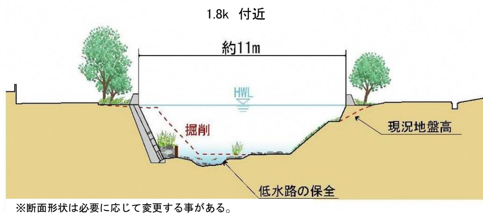
図 4-11 大沢川横断イメージ
