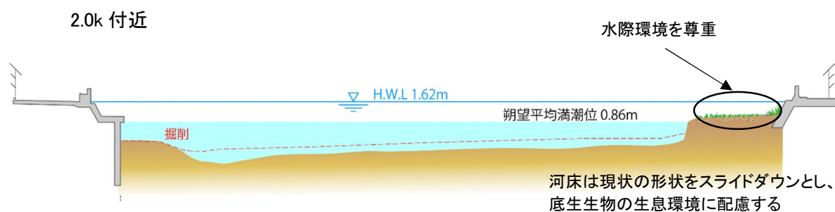
図 4-8 改修横断イメージ図
