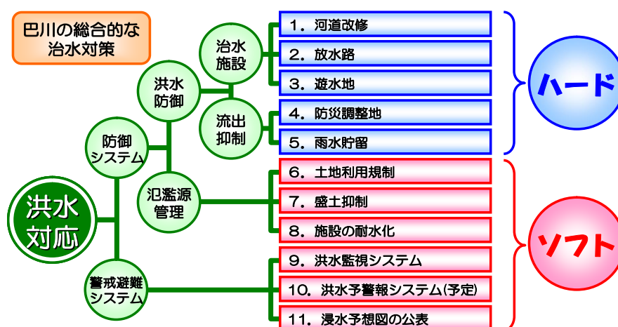
図 2-7 総合的な治水対策システム
