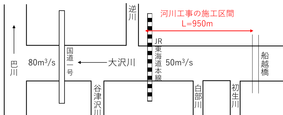
図 4-10 流量配分図
