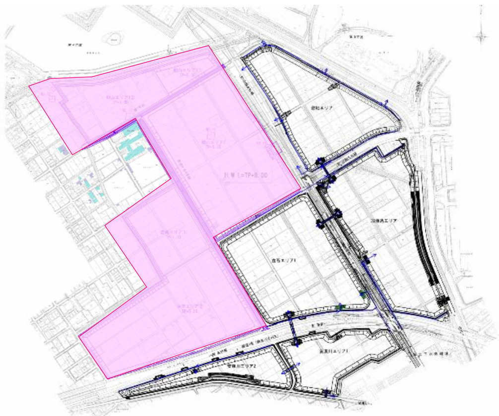
図 4-4 麻機遊水地第2工区平面図
