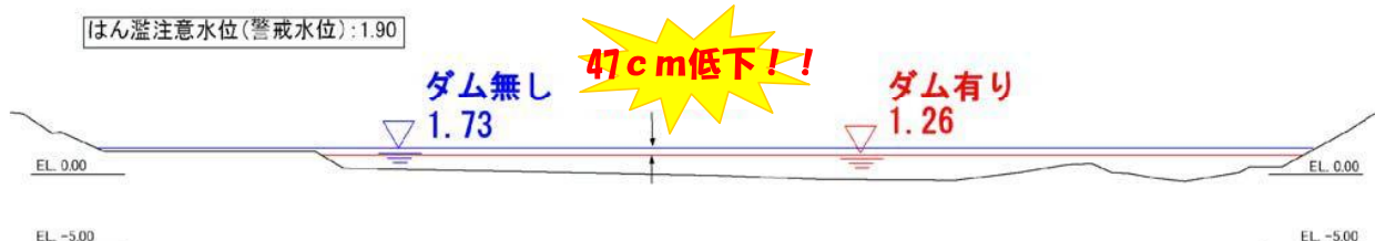
天方水位観測局 横断面図
