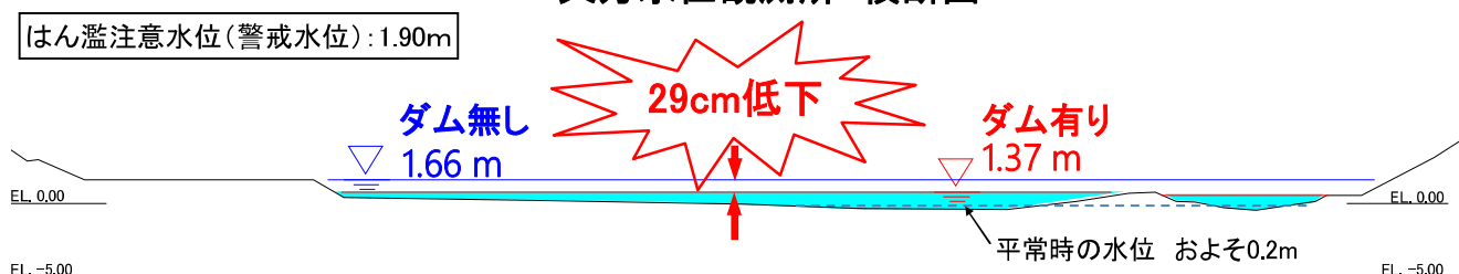
10月12日 ダムの洪水低減効果(天方観測所)
