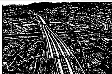
写真3 静岡BP清水立体高架化工事
