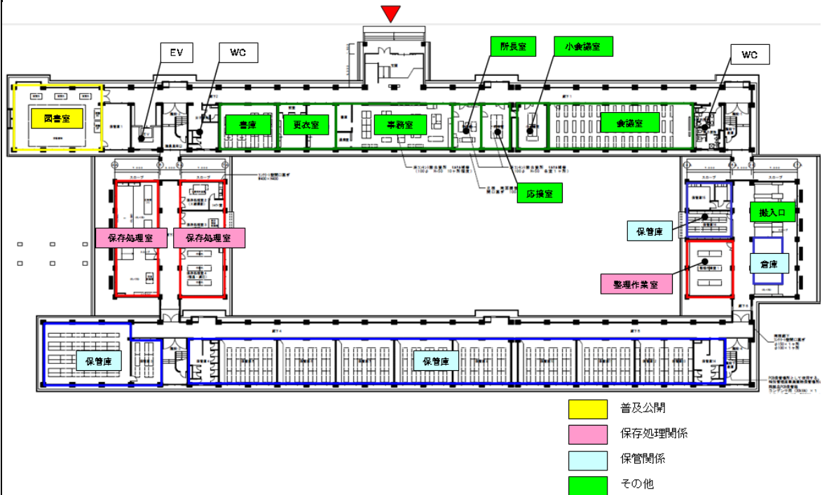
1階平面図
